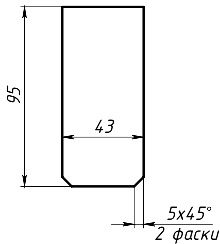
Поз.2 (Ребро)
